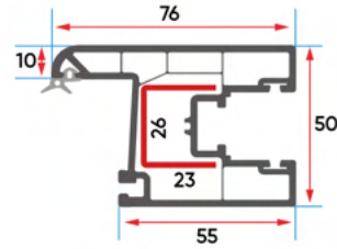
S 1019 Sürme Kanat Sliding Window Sash
