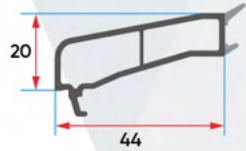
ER 7015 Süper Tek Cam Çıtası Super Single Glazing Bead
