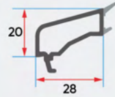
ER 7016 Süper Çift Cam Çıtası Super Double Glazing Bead
