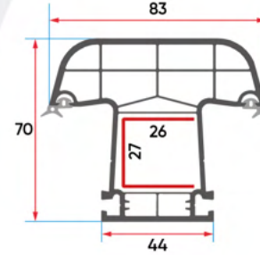
ER 7019 Oval Orta Kayıt Profili Ovoid Mullion Profile
