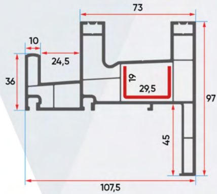
S 1020 Sürme Sineklik Pervazlı Kasa Profili Sliding Screen Frame with Cornice Profile
