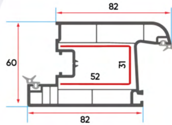
ER 6025 Oval Kapı Kanat Profili Ovoid Door Sash Profile
