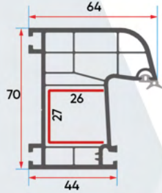
ER 7018 Oval Kanat Profili Ovoid Frame Profile
